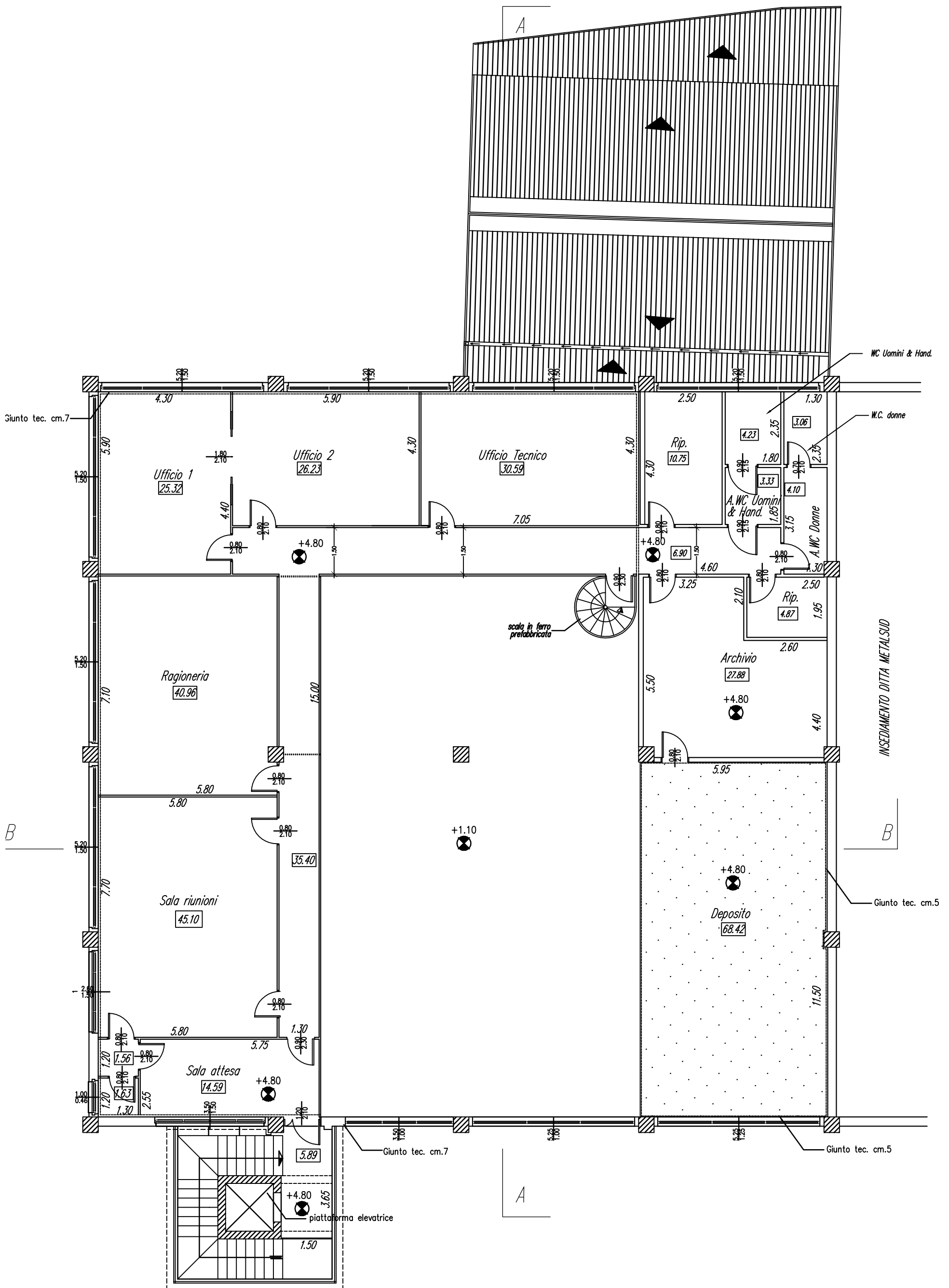
PIANTA PIANO SOPPALCATO QUOTA + 4.80 Scala 1:100
